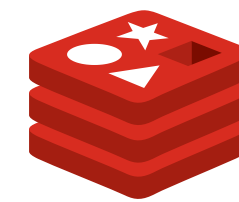
Redis
