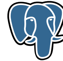
Postgres
